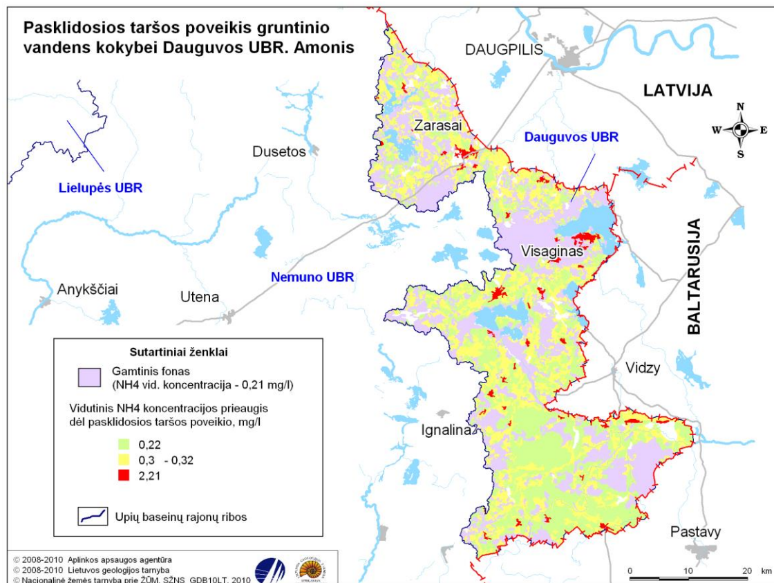
2.11 pav. Pasklidusios taršos poveikis gruntinio vandens kokybei. Amonis.
