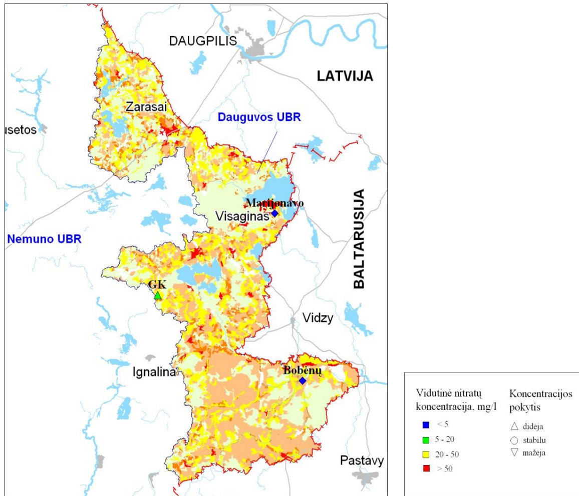
2.10 pav. Pasklidusios taršos poveikis gruntinio vandens kokybei. Nitratai.
